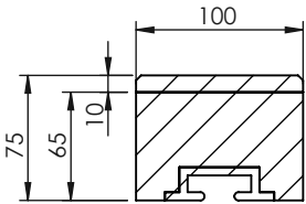
SEZIONE A-A
