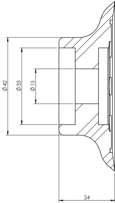
SEZIONE A-A
