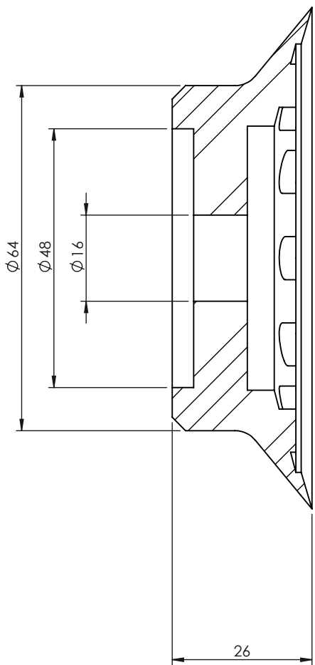
SEZIONE A-A
